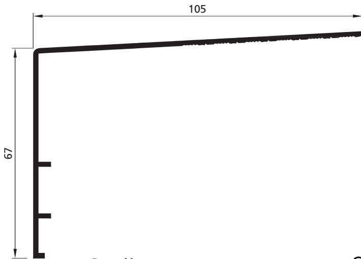
Cornières d'habillage
