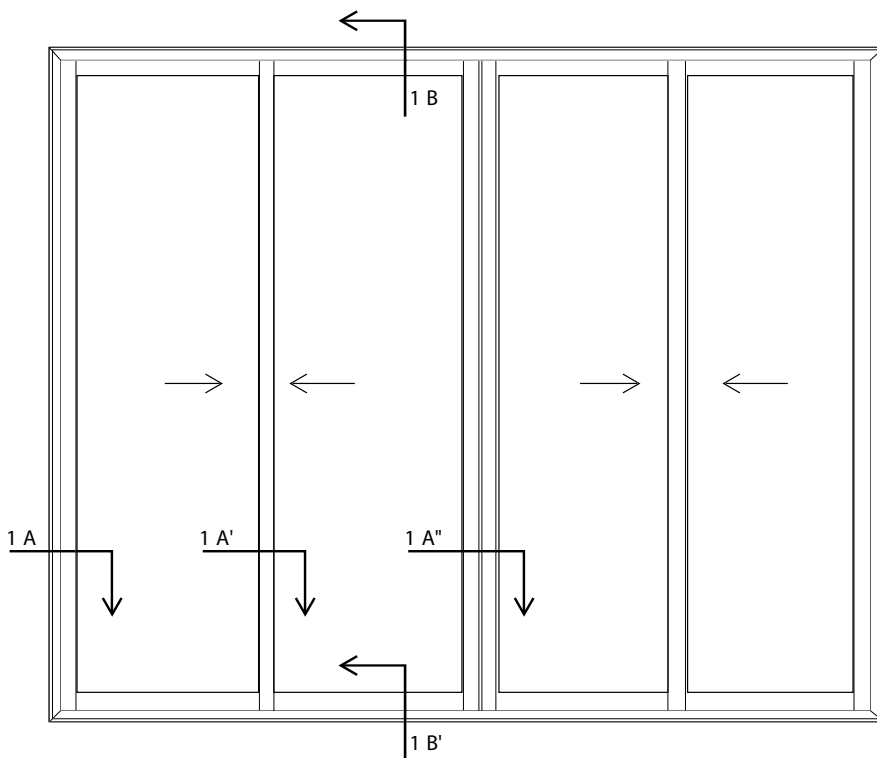
Porte-fenêtre coulissante, 4 vantaux sur 2 rails (vue de l'extérieur)
