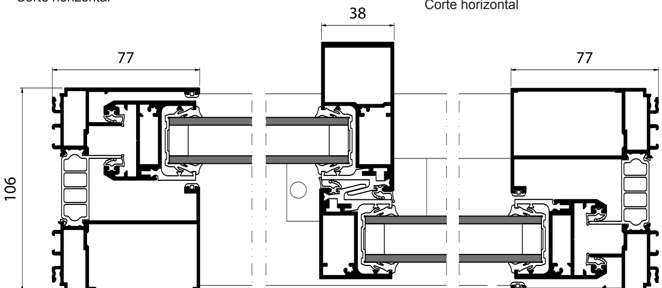
Coupe horizontale Horizontal cross section Corte horizontal
