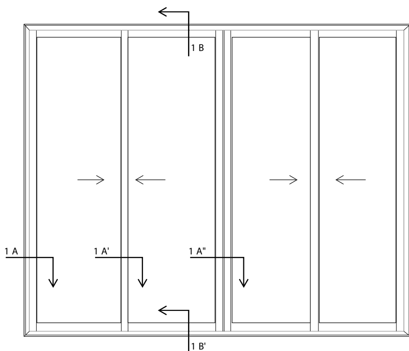
Porte-fenêtre coulissante, 2 vantaux (vue de l'extérieur) Sliding patio-door, 2 leaves (outside view) Corredera, 2 hojas (vista externa)
