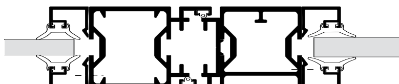
Coupe horizontale 1B Horizontal cross section Corte horizontal
