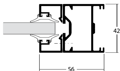
Coupe horizontale 1C Horizontal cross section Corte horizontal
