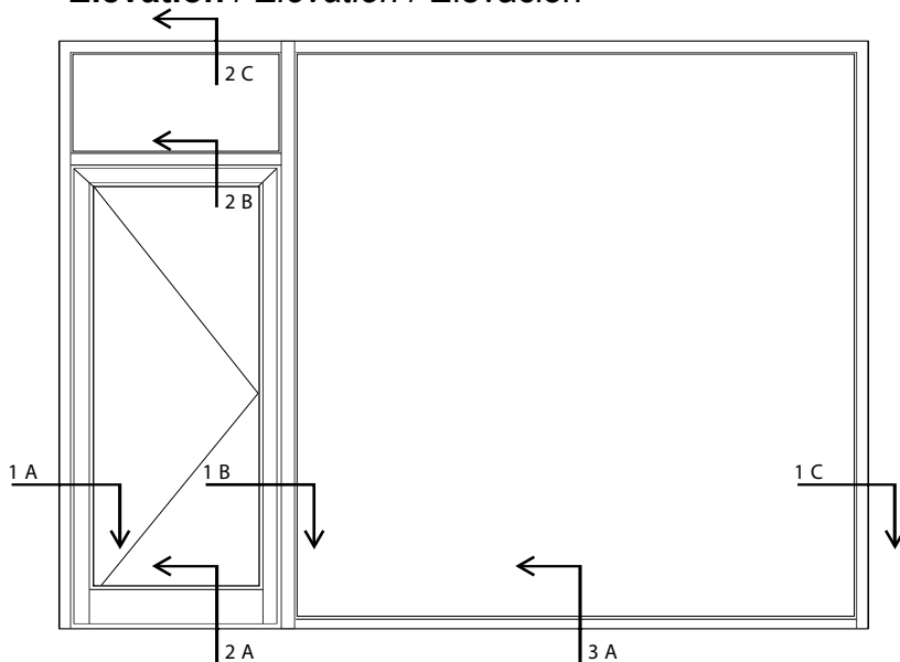
Devanture avec porte 1 vantail et imposte Shop front with 1-leaf door and top fixed light Escaparate con puerta 1 hoja y fijo superior
