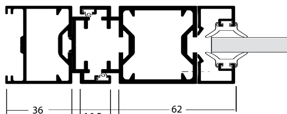
Coupe horizontale 1A Horizontal cross section Corte horizontal
