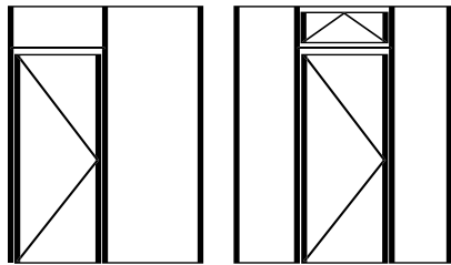
Porte 1 vantail sous imposte fixe ou à soufflet avec fixe(s) latéral(aux) 1-leaf door with top and lateral fixed light(s) or bottom hung fanlight Puerta 1 hoja con fijo superior y lateral o abatible superior y fijos laterales
