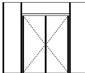
Porte 2 vantaux sous imposte avec fixes latéraux (ouv. ext) 2-leaf door with top and side fixed lights (outward opening) Puerta 2 hojas con fijos superior y laterales (apertura al exterior)
