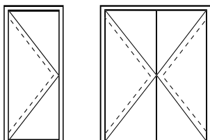
Porte 1 et 2 vantail 1 & 2-leaf door Puerta 1 y 2 hojas
