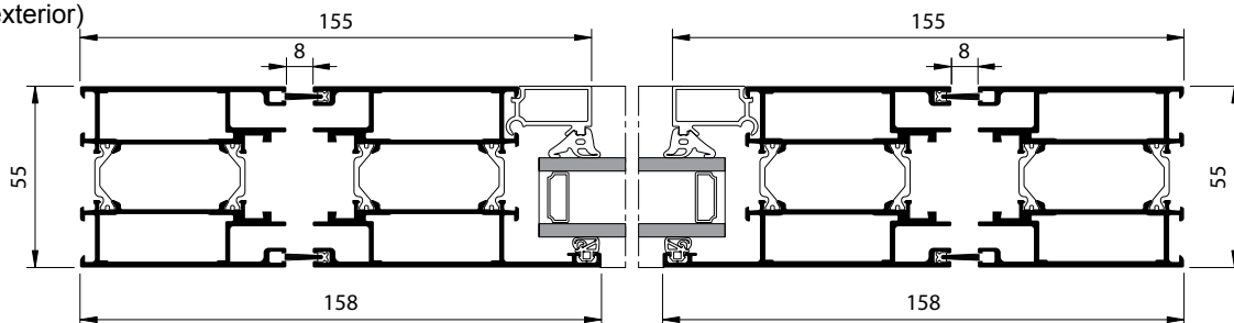
Porte 2 vantaux (vue de l'ext.) 2-leaf door (outside view) 2 hojas (apertura al exterior)
