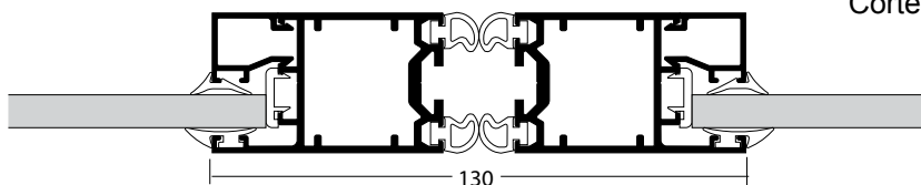
Coupe horizontale 1C - B Horizontal cross section / Corte horizontal
