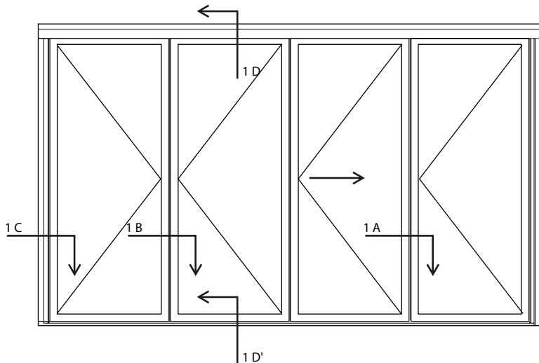
Porte 4 vantaux ouverture vers l'intérieur (vue de l'extérieur) 4-leaf door inward opening (external view) Puerta 4 hojas apertura al interior (vista externa)
