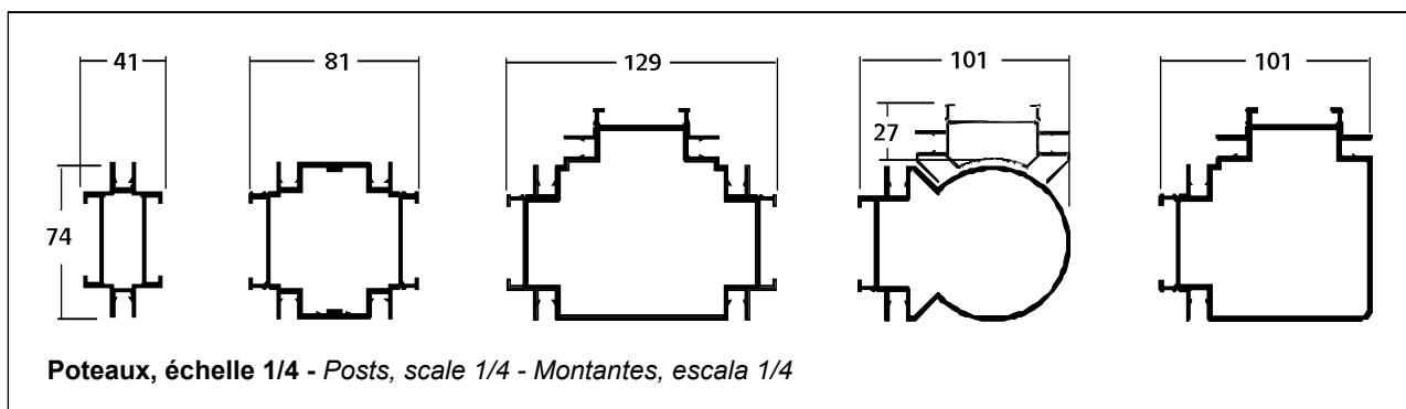
Coupe horizontale, départs en angle variable de 90 à 180° Horizontal cross-section, 90° to 180° adjustable angle posts Corte horizontal, départs en angle variable de 90 à 180°
