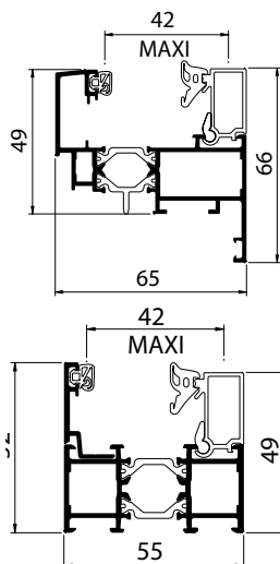
Prise de volume Infill volume Acristalamiento
