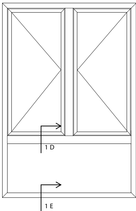
Châssis à la française 2 vantaux (vue de l'ext.)
