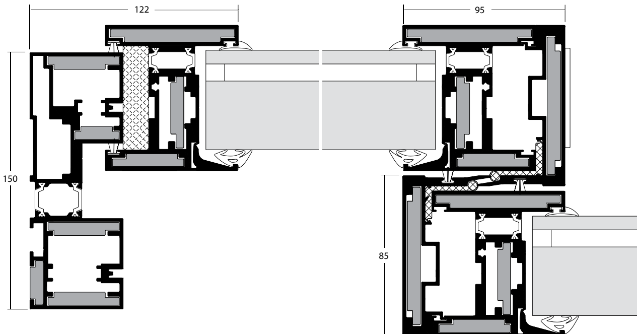
Coupe horizontale 1A - A' Horizontal cross section Corte horizontal
