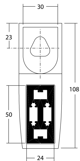
Coupe horizontale 1A Horizontal cross section Corte horizontal
