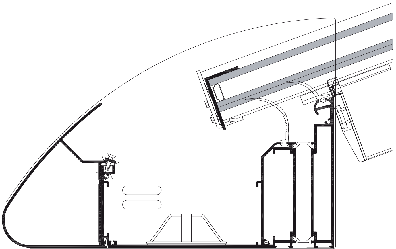
Coupe verticale, sablière
