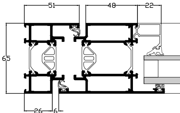
Coupe horizontale 1 B-B'
