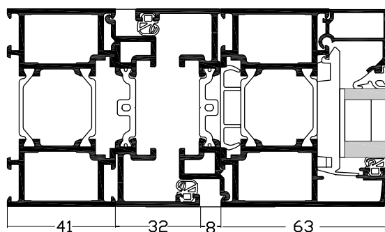
Coupe horizontale 1 A
