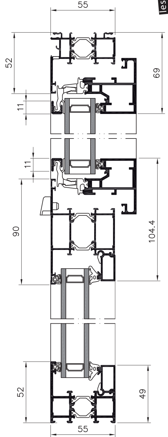
Coupe verticale 1 D - E
