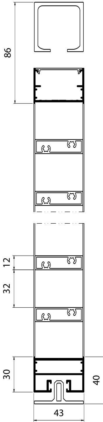
Coupe verticale
