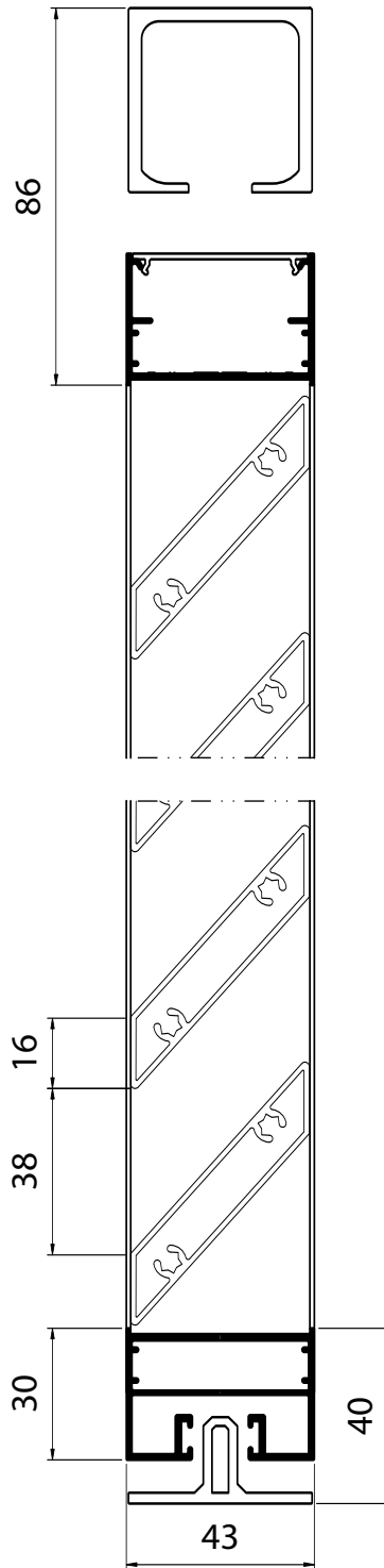
Coupe verticale
