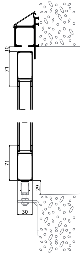
Coupe verticale
