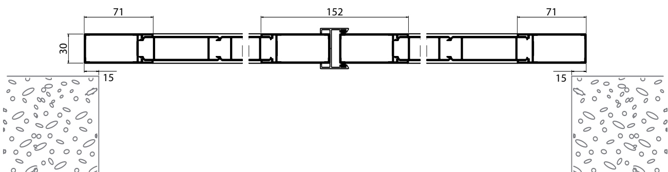
Coupe horizontale
