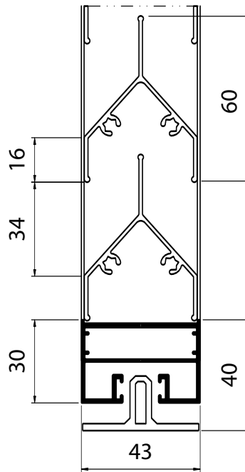
Coupe verticale
