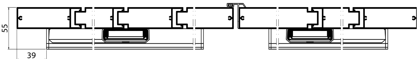
Coupe horizontale
