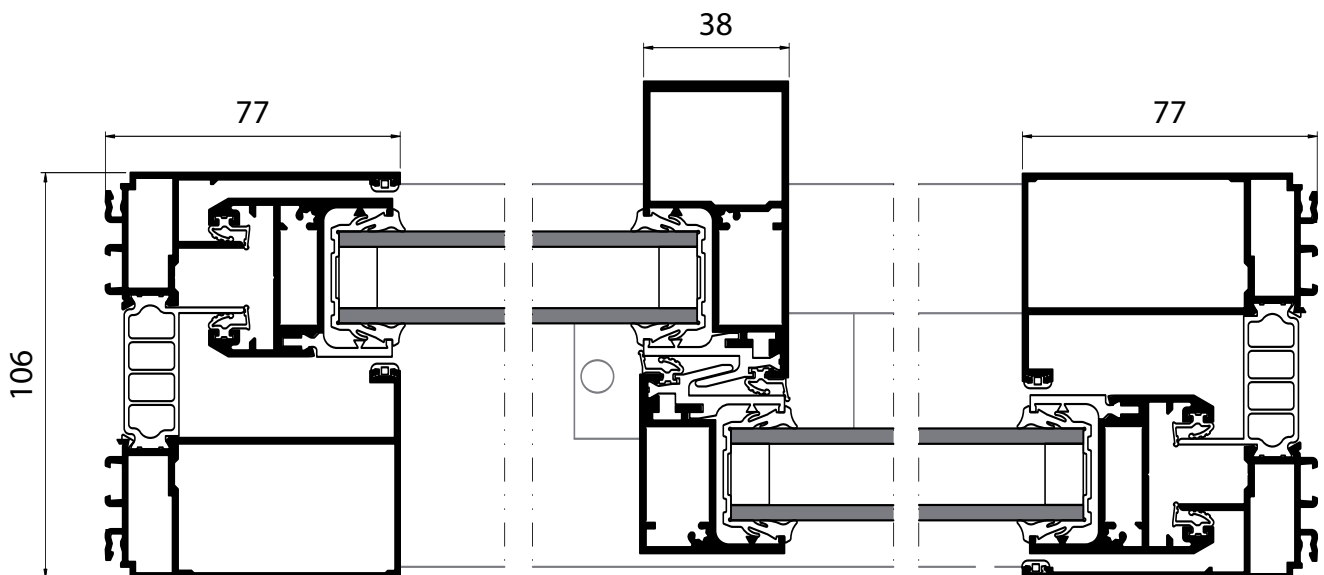
Coupe horizontale
