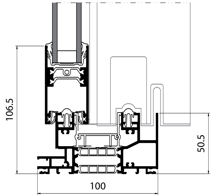
Coupe verticale
