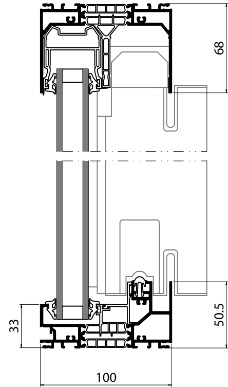
Coupe verticale
