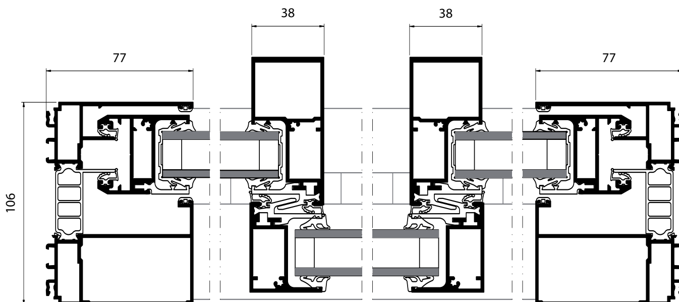
Coupe verticale
