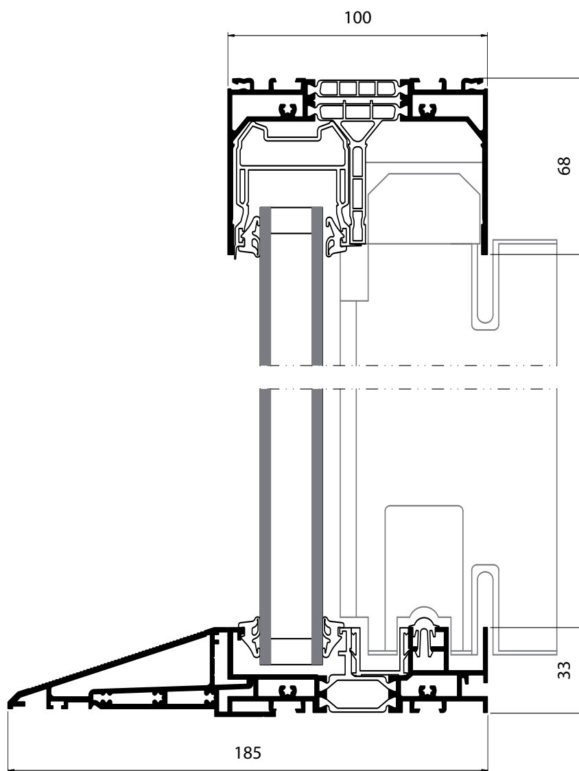
Coupe verticale
