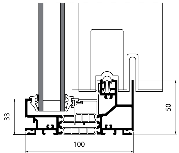
Coupe verticale
