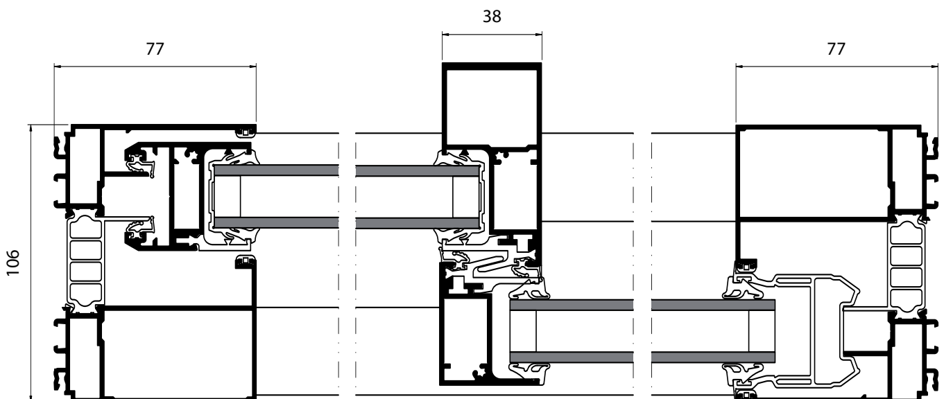
Coupe horizontale
