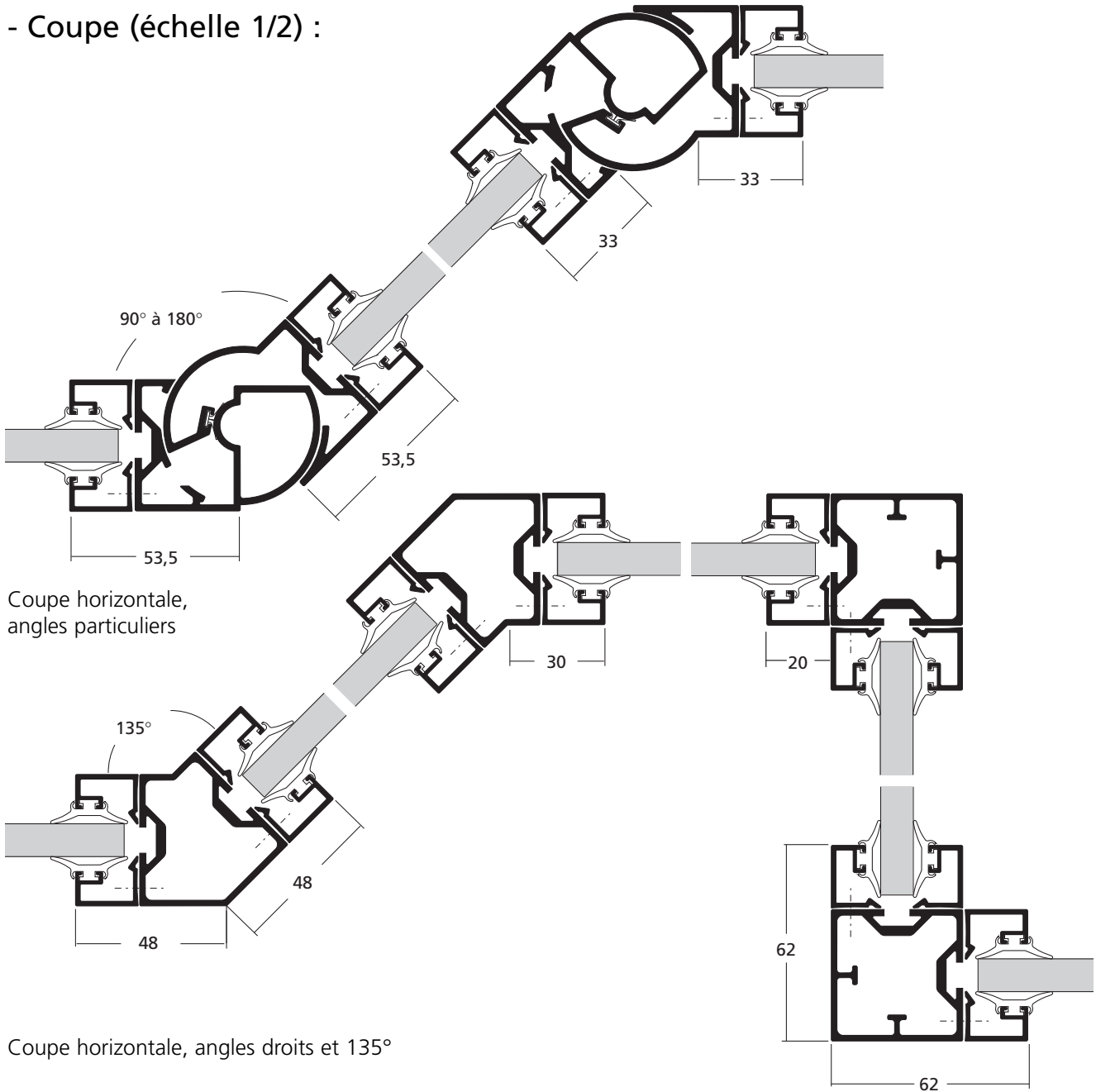
Devanture avec retrait (angles 135° et 90°)
