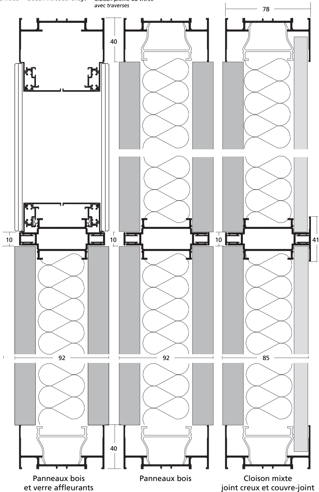
Cloison vitrée sur allège
