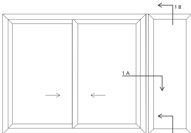
Fenêtre 2 vantaux + fixe latéral (vue de l'extérieur)
