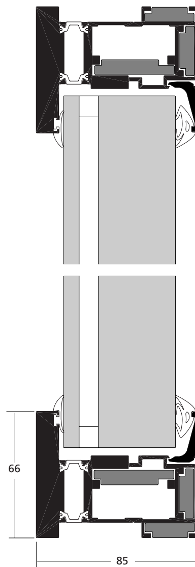
Coupe verticale 1 B - B'
