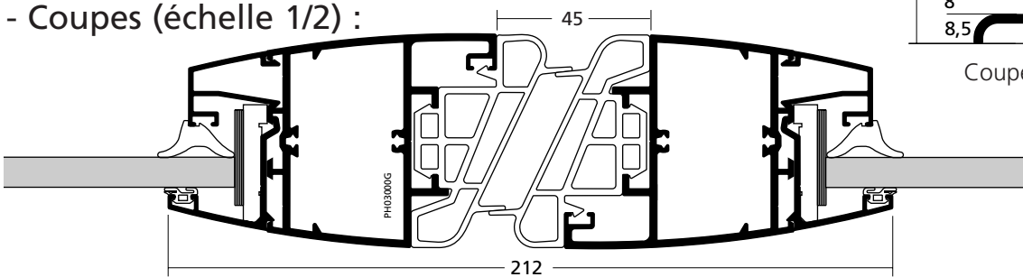
Coupe horizontale 1 B
