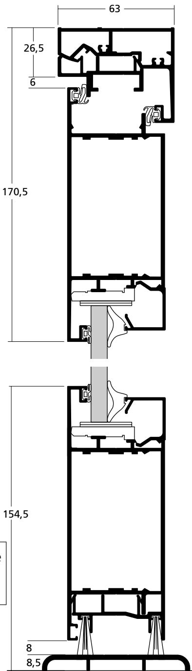
Coupe verticale 1 C - C'
