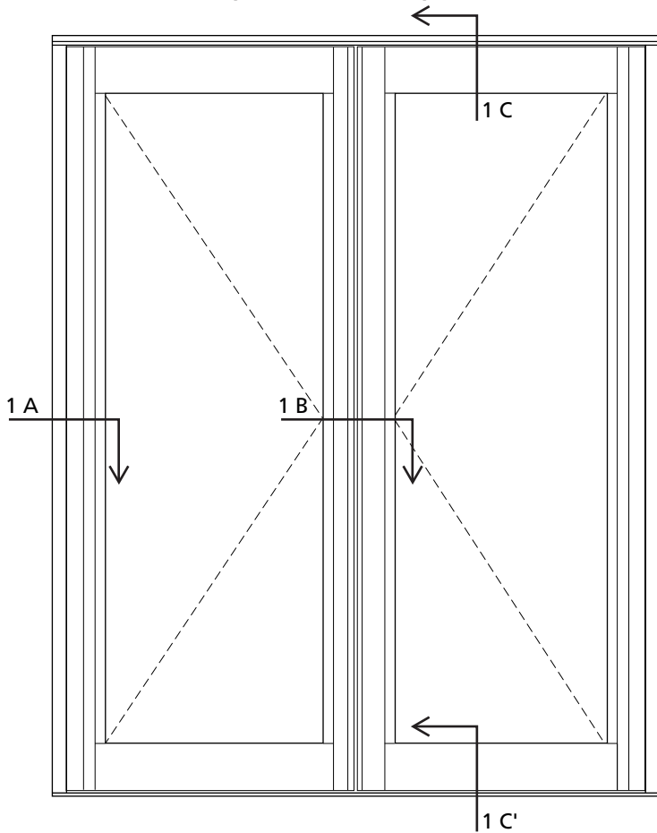
Porte 2 vantaux (vue de l'extérieur)
