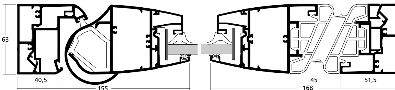
Coupe horizontale 1 A
