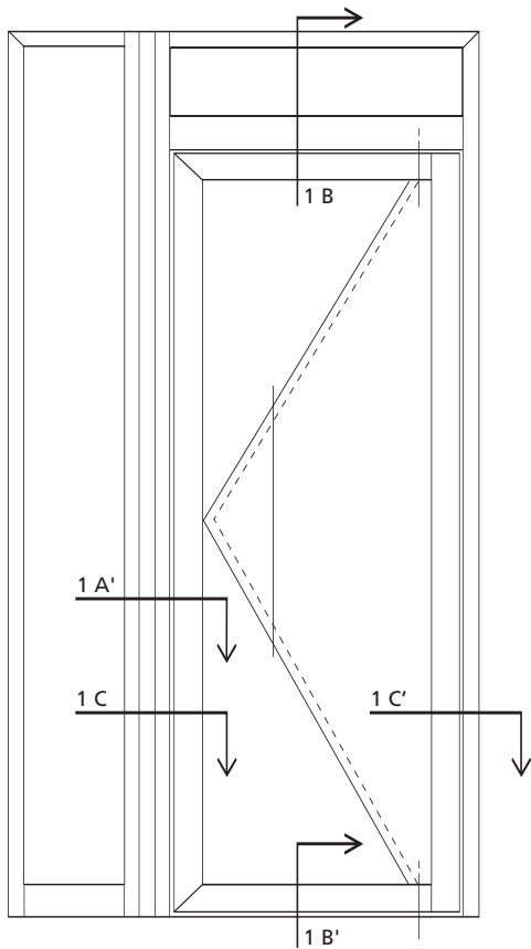
Porte 1 vantail avec imposte et fixe latéral (vue de l'extérieur)
