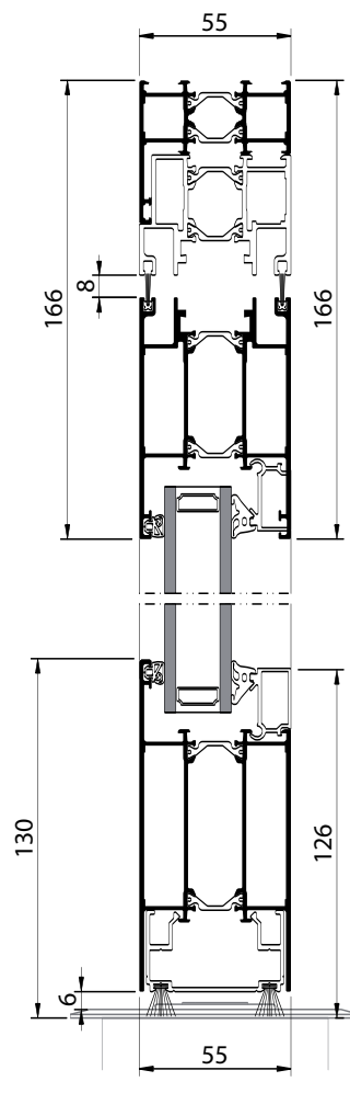
Coupe verticale 1 B - B'
