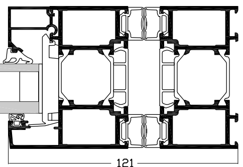
Coupe horizontale 1 B B'
