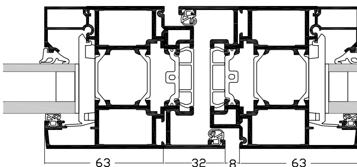
Coupe horizontale 1 A
