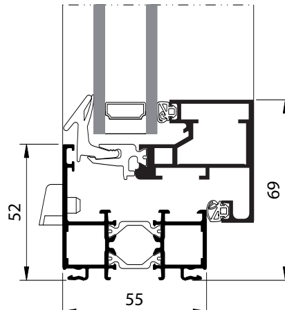
Coupe verticale 1 D - E
