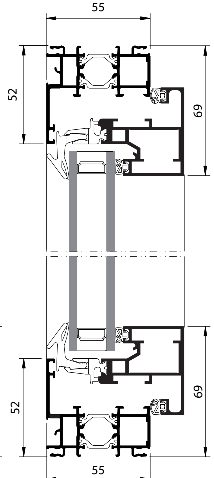
Coupe verticale 1 D - E Drainage caché
