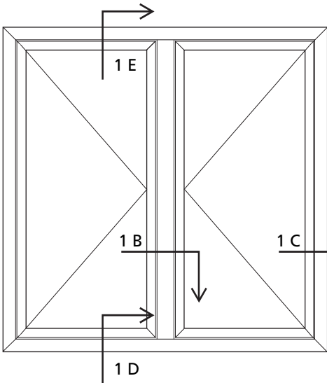
Châssis à la française 2 vantaux (vue de l'extérieur)
