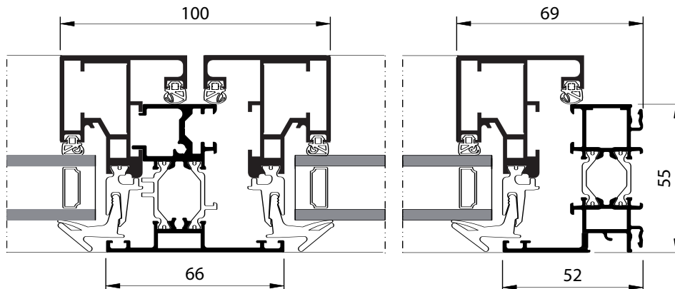
Coupe horizontale 1 B - C
