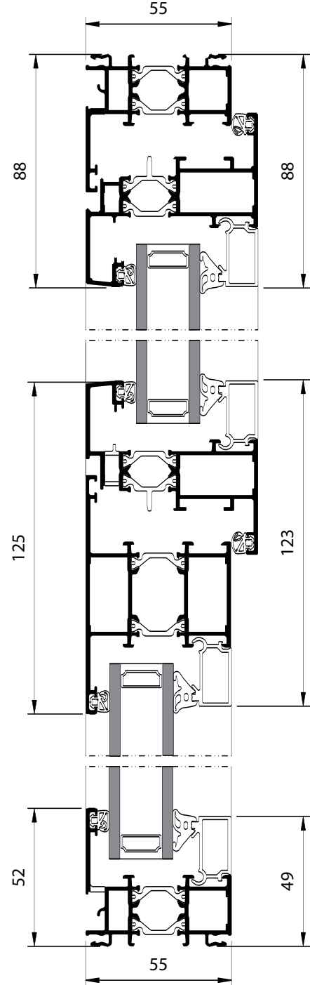
Coupe verticale 1 D - E (Drainage caché traverse)
