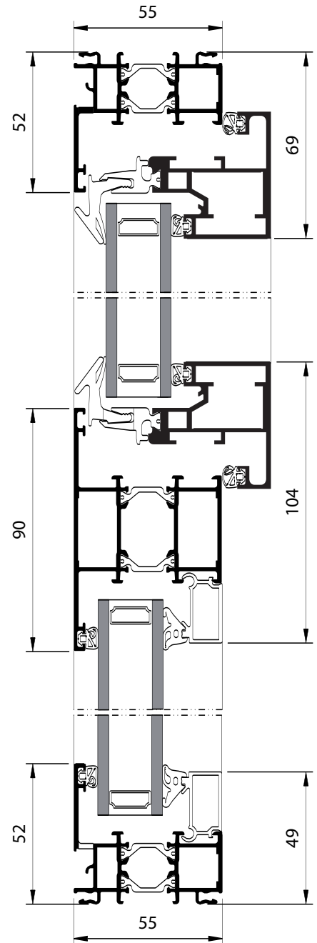
Coupe verticale 1 D - E (Drainage caché traverse)
