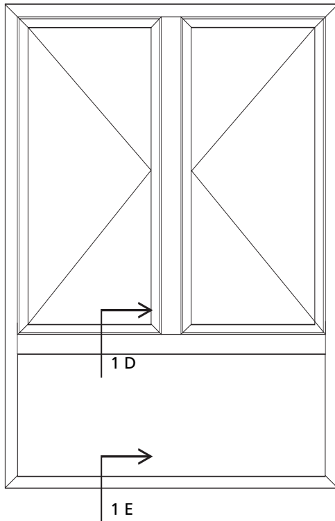
Châssis à la française 2 vantaux sur allège (vue de l'extérieur)
