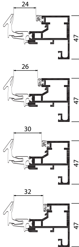
Parclose chant clipable
