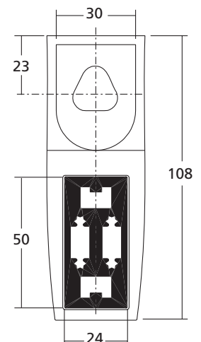
Coupe horizontale 1-A
