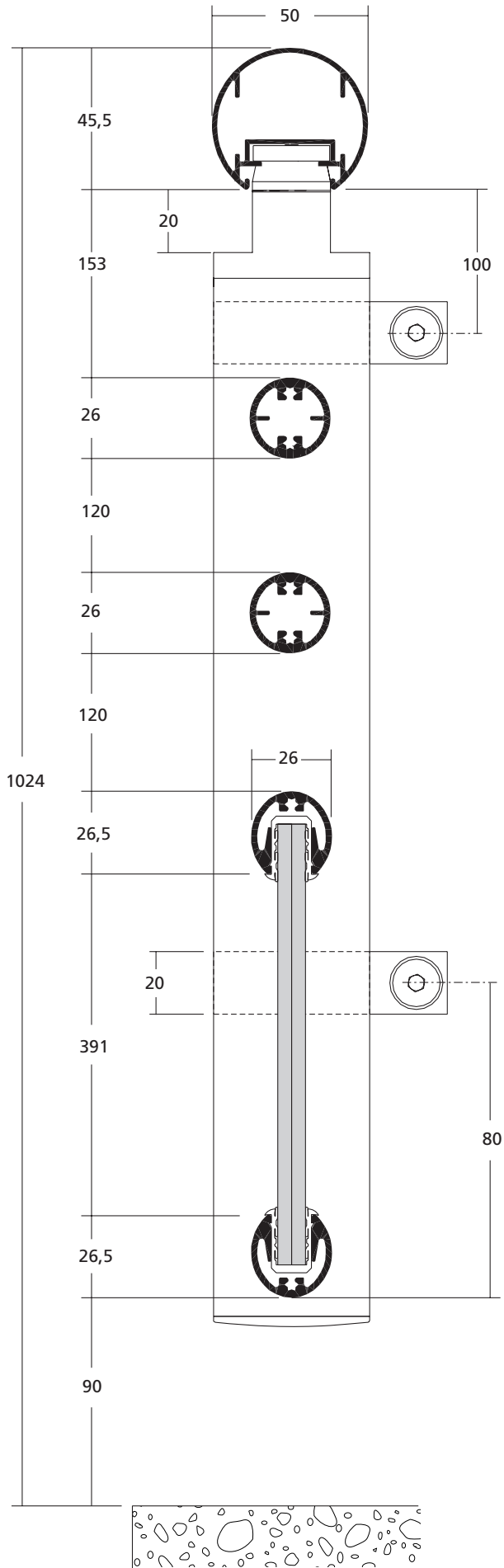
Coupe verticale 1-B
