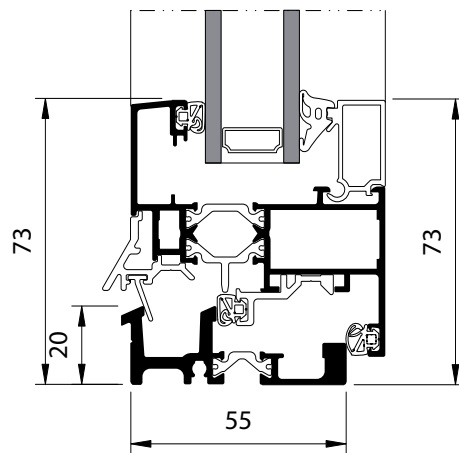
Ouvrant apparent Coupe verticale 1 C - D
