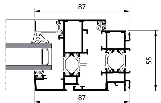
Coupe horizontale 1 A
