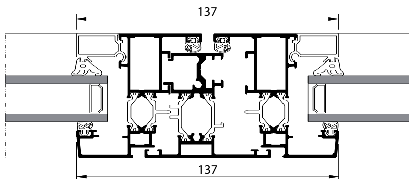
Coupe horizontale 1 B
