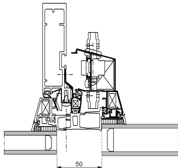
Coupe supérieure 1C
